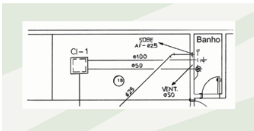
Projeto de esgoto sanitário do banheiro.
